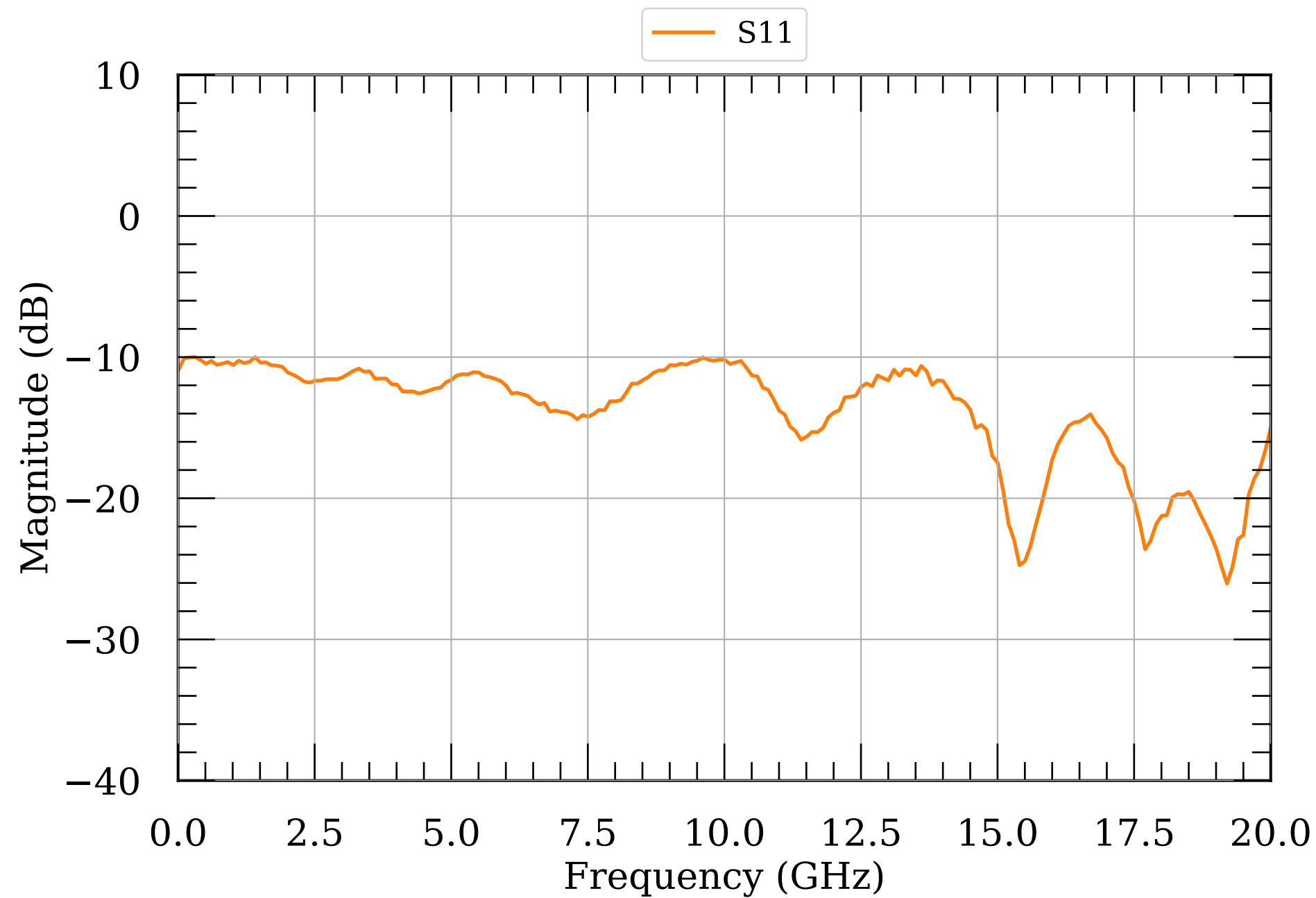
LNA S-params module026
